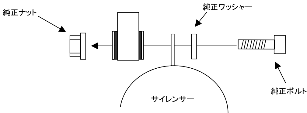
車体後方から見た図です。模式図の為、ボルト・ナット等の形状が実際とは異なります
