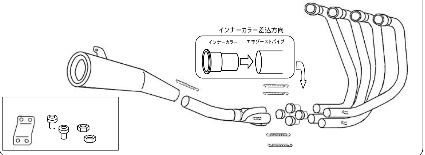
パーツリスト(梱包内容)
