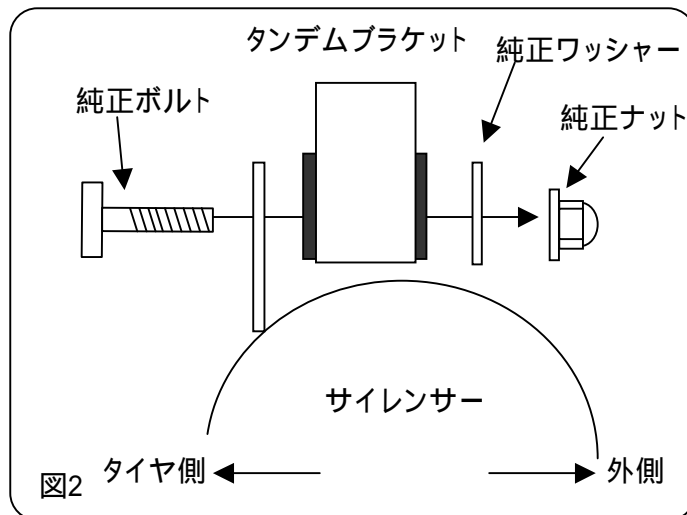
模式図の為、ボルト・ナット等の形状が実際とは異なります。
